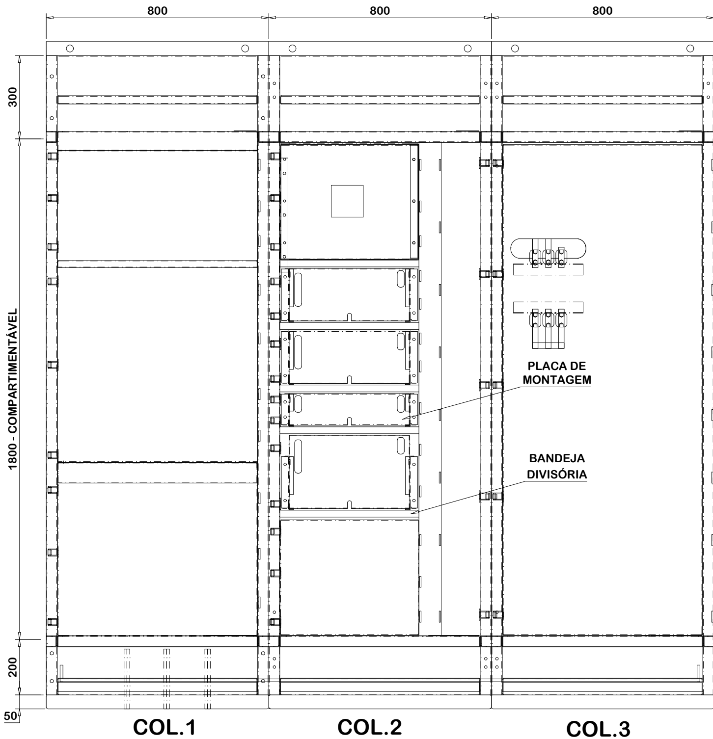
VISTA FRONTAL S/ PORTAS E S/ TAMPAS
