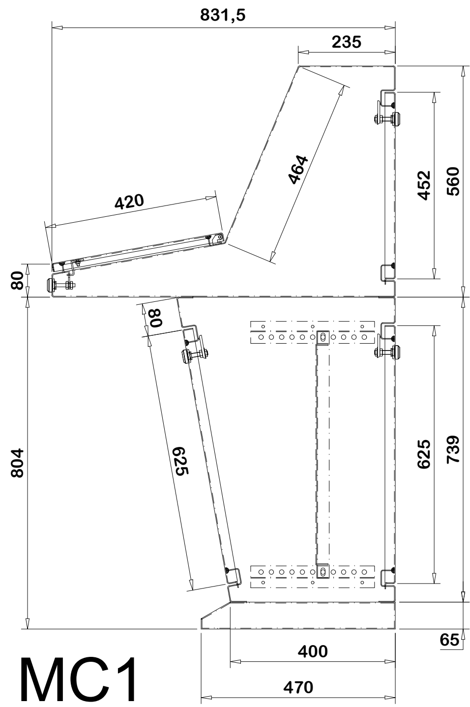
VISTA LATERAL
