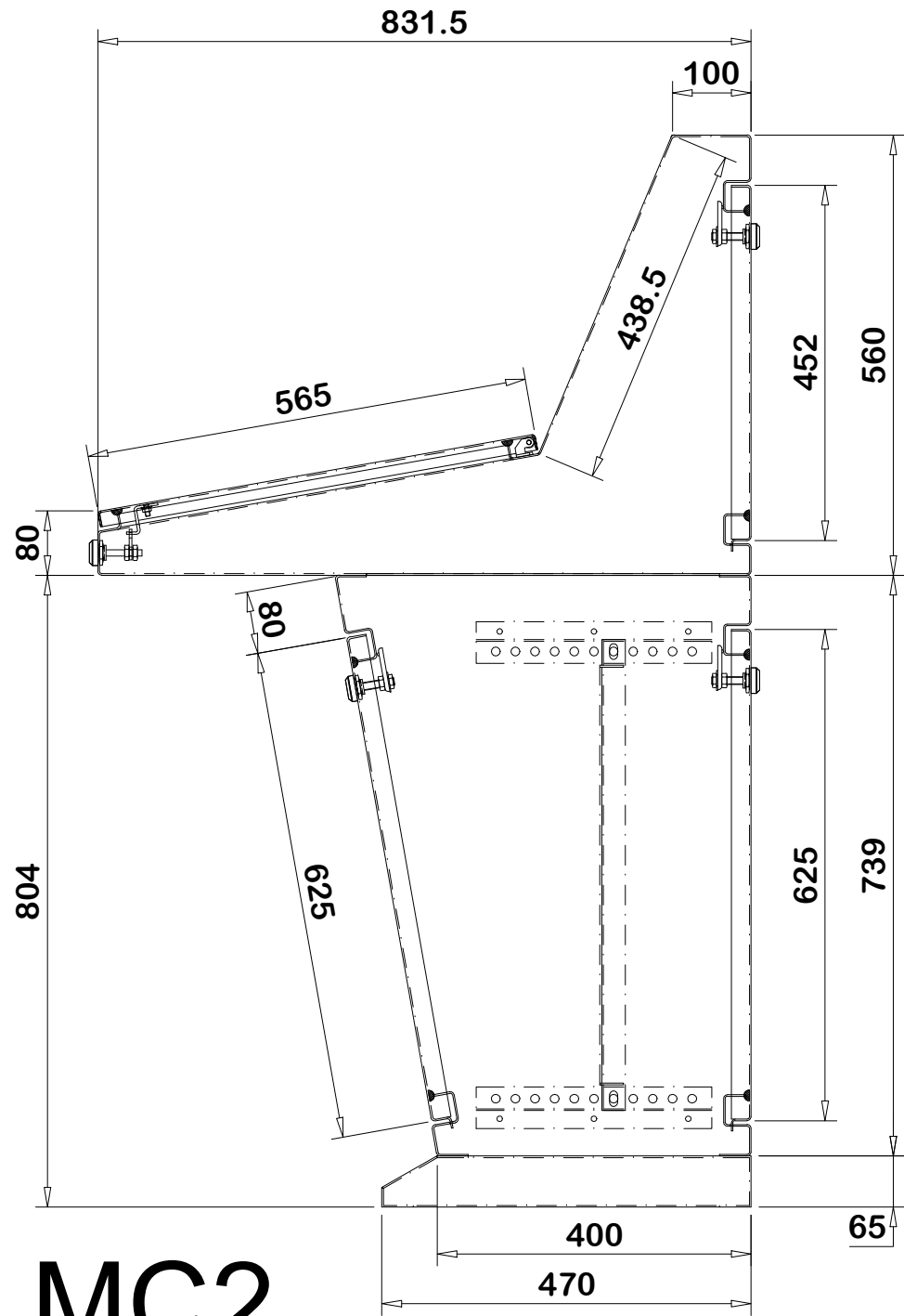
VISTA LATERAL
