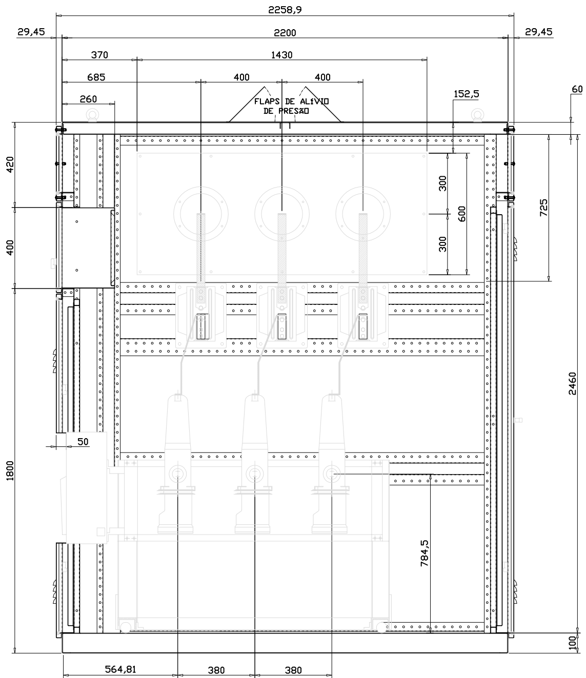
CORTE "CC"
