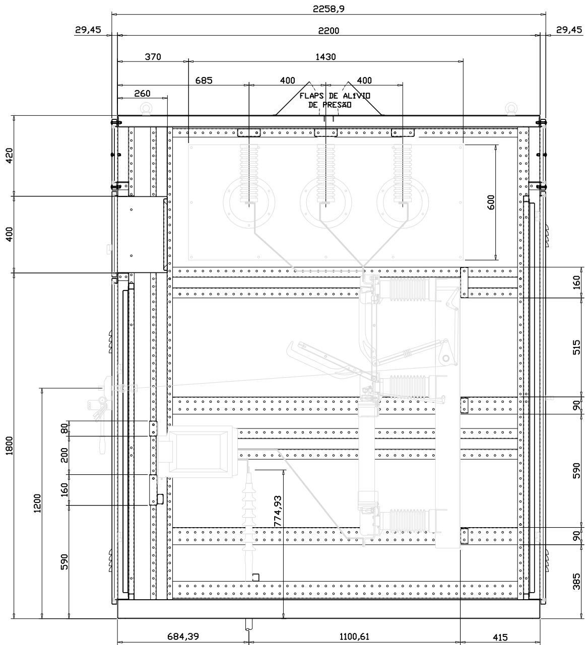
CORTE "DD"
