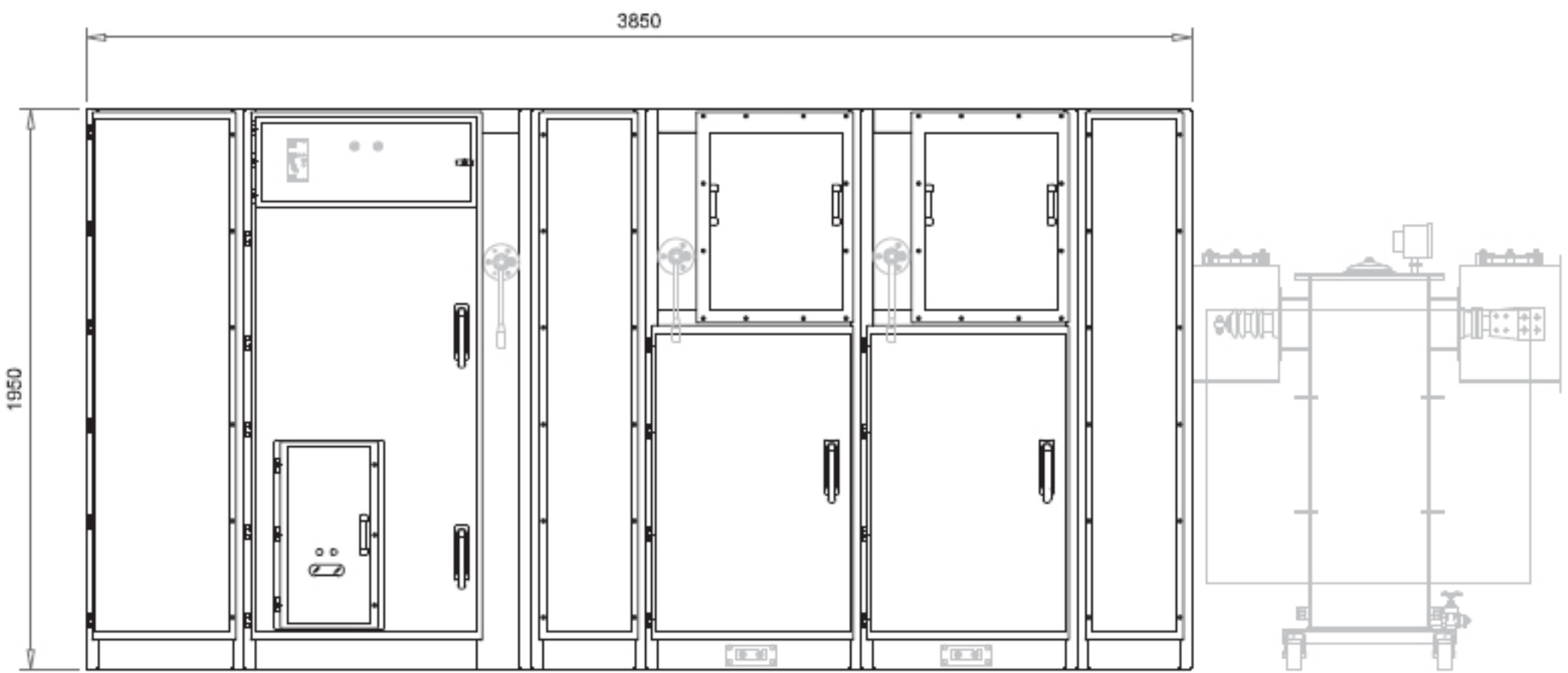
VISTA FRONTAL COM PORTA
