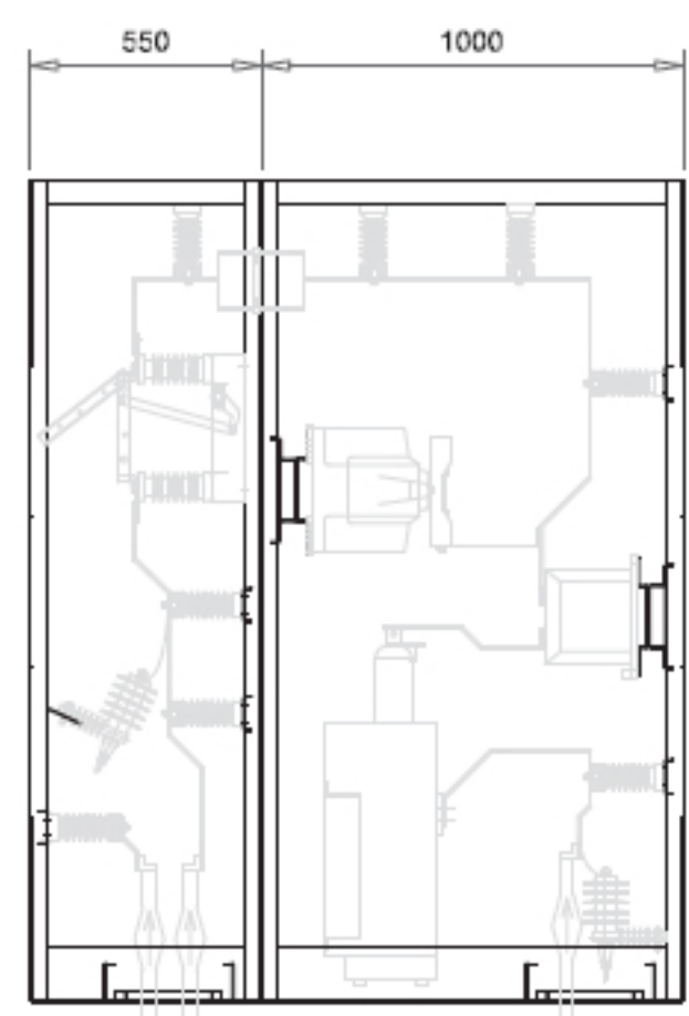
ENTRADA COM CHAVE DISJUNTOR SAÍDA COM CABO VISTA FRONTAL SEM PORTA
