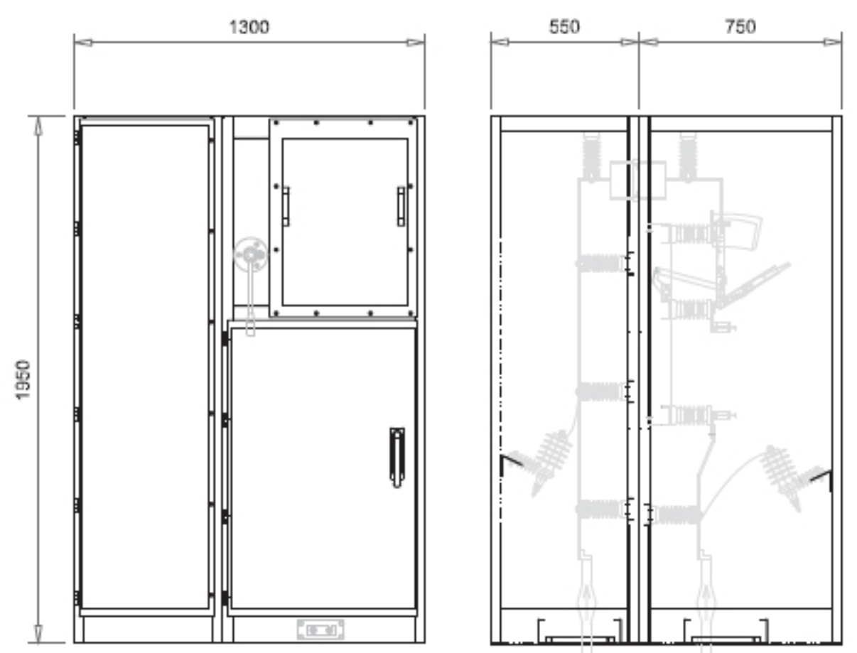
VISTA FRONTAL COM PORTA
