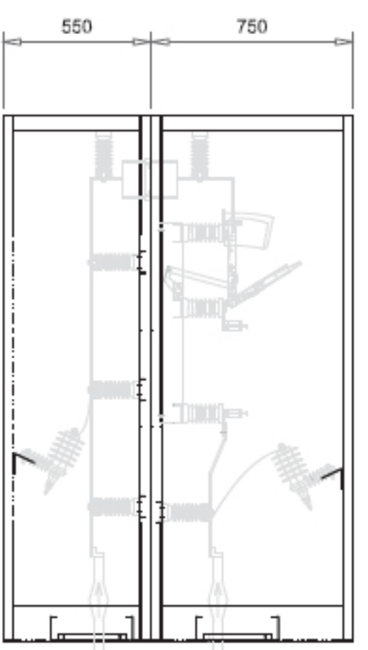
ENTRADA CHAVE SECCIONADORA VISTA FRONTAL SEM PORTA
