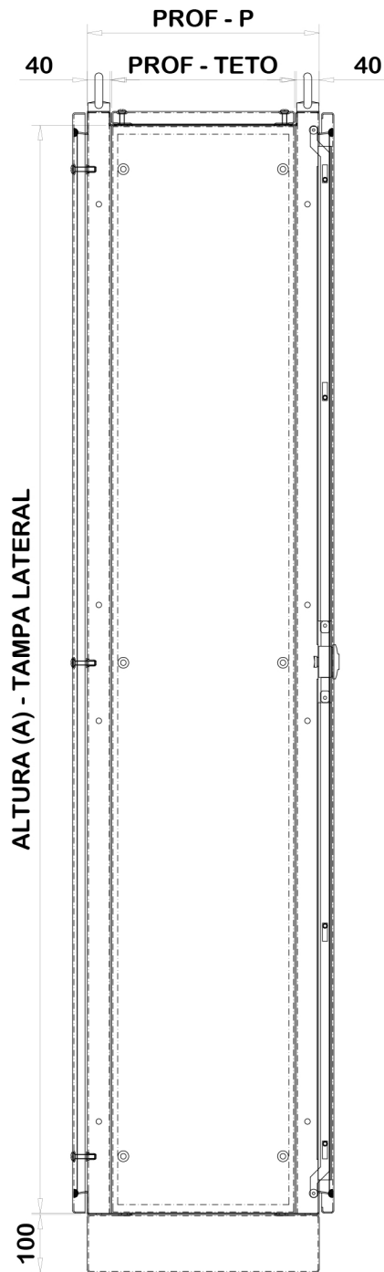
VISTA LATERAL
