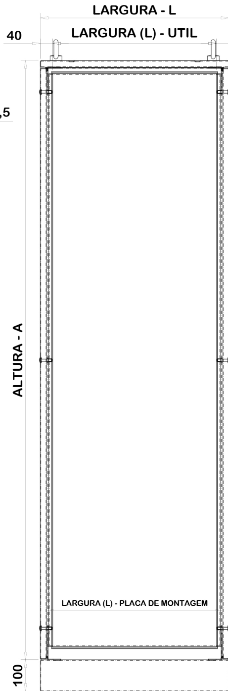
VISTA FRONTAL SEM PORTA
