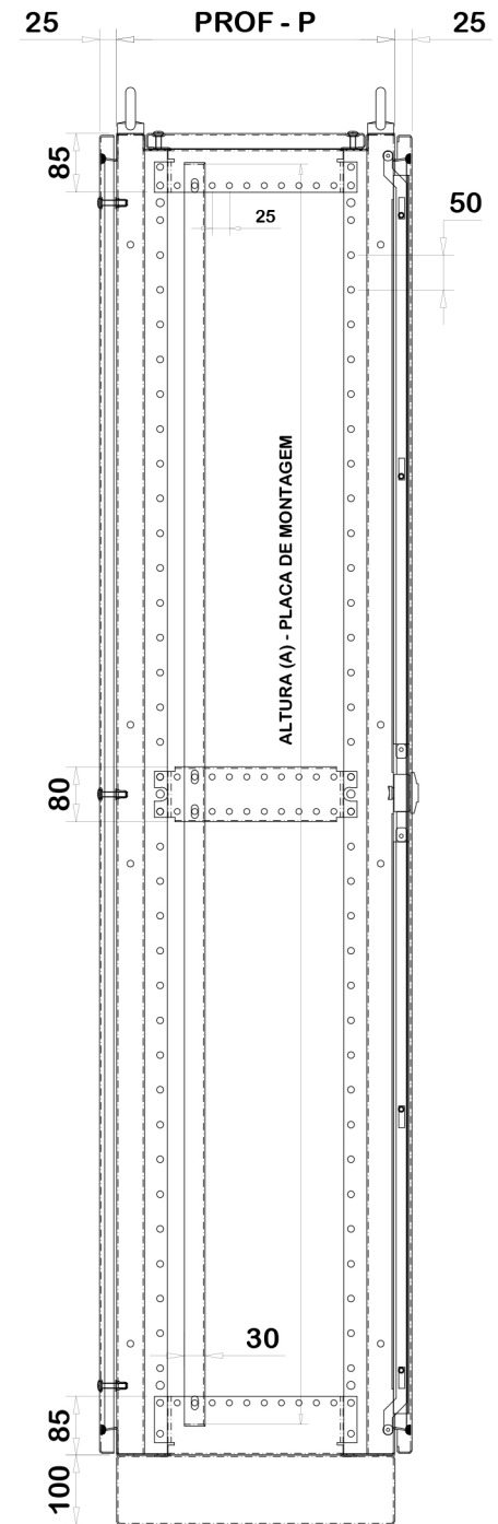
VISTA LATERAL SEM TAMPA
