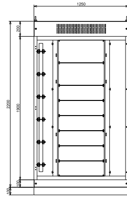
FRONTAL SEM PORTA EXTERNA
