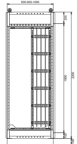
LATERAL OPÇÃO 2 (DD) (BARRAMENTO LATERAL)
