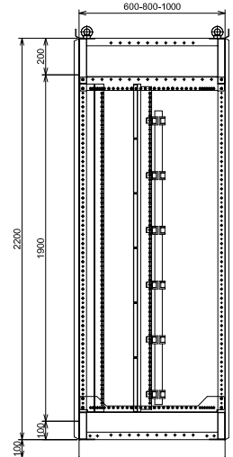
LATERAL OPÇÃO 1 (BB) (BARRAMENTO TRASEIRO)
