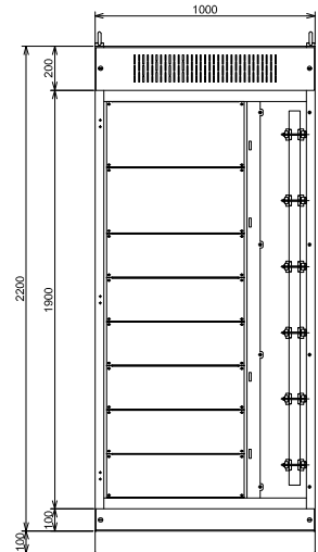
FRONTAL SEM PORTA EXTERNA
