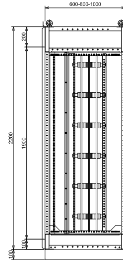
LATERAL OPÇÃO 2 (BARRAMENTO LATERAL)
