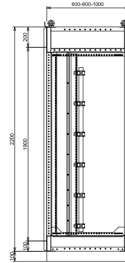
LATERAL OPÇÃO 1 (BARRAMENTO TRASEIRO)
