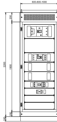
FRONTAL SEM PORTA
