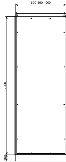
VISTA TRASEIRA / LATERAL
